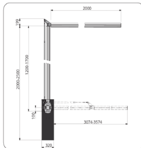
Articulación para asta elíptica
