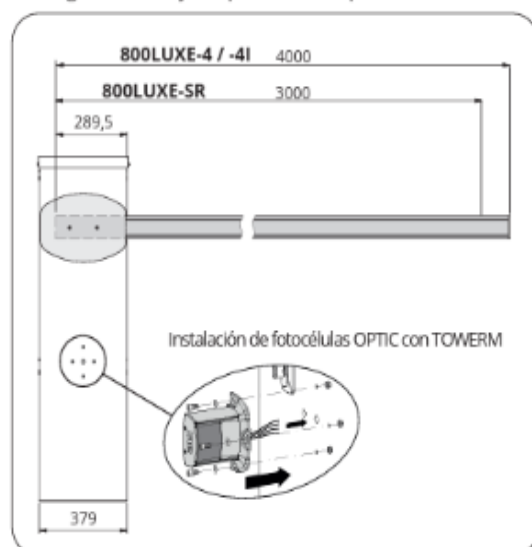
Longitud del asta y compartimento de paso
