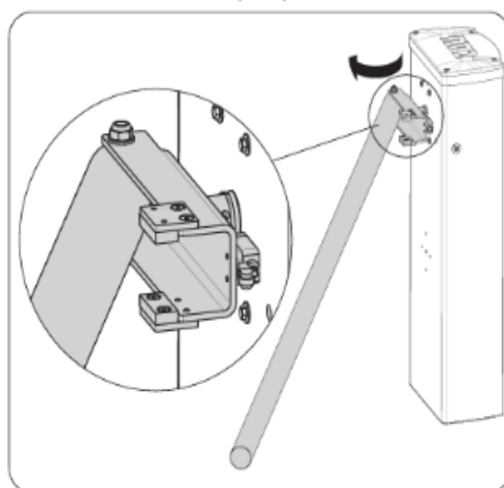
Sistema de rotura en caso de impacto para asta redonda (P-800SFA)
