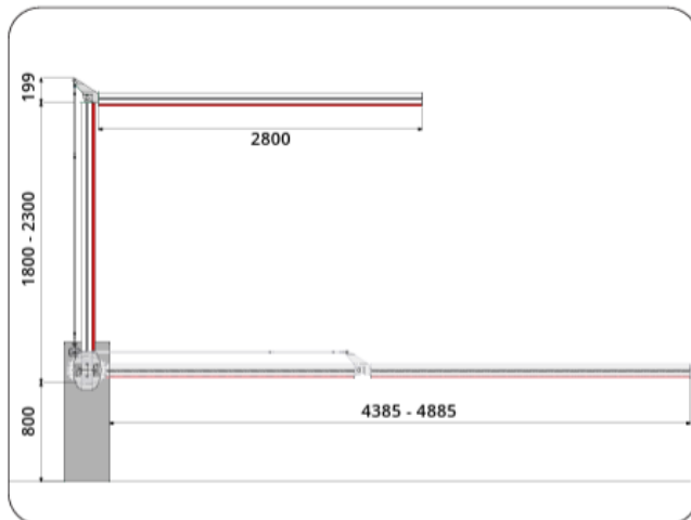
Longitud del asta elíptica y compartimento de paso
