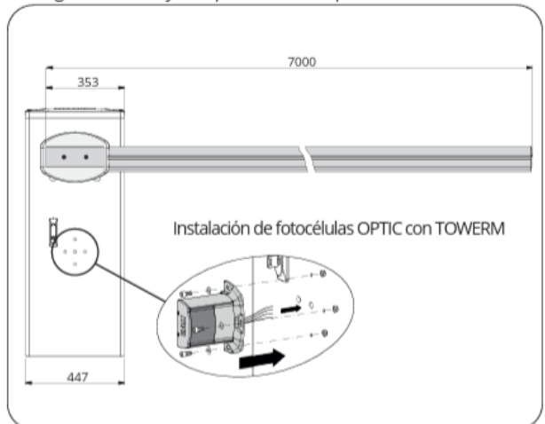
Longitud del asta y compartimento de paso
