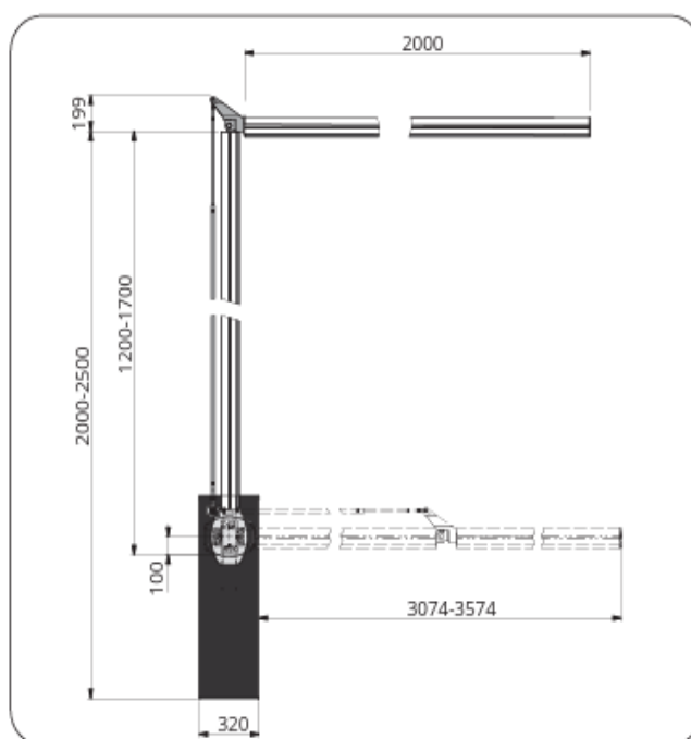
Articulación para asta elíptica
