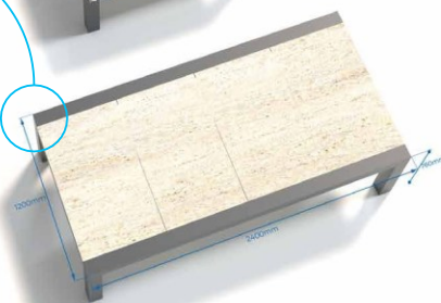
Gran gusto E Con placas 600 mm Con painéis 600 mm 2400x1200x760 mm
