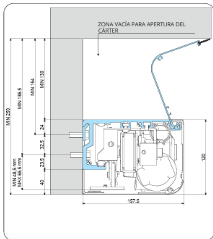
Dimensiones mínimas para abrir la carcasa hacia arriba
