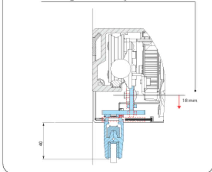
Rango máximo de ajuste del carro
